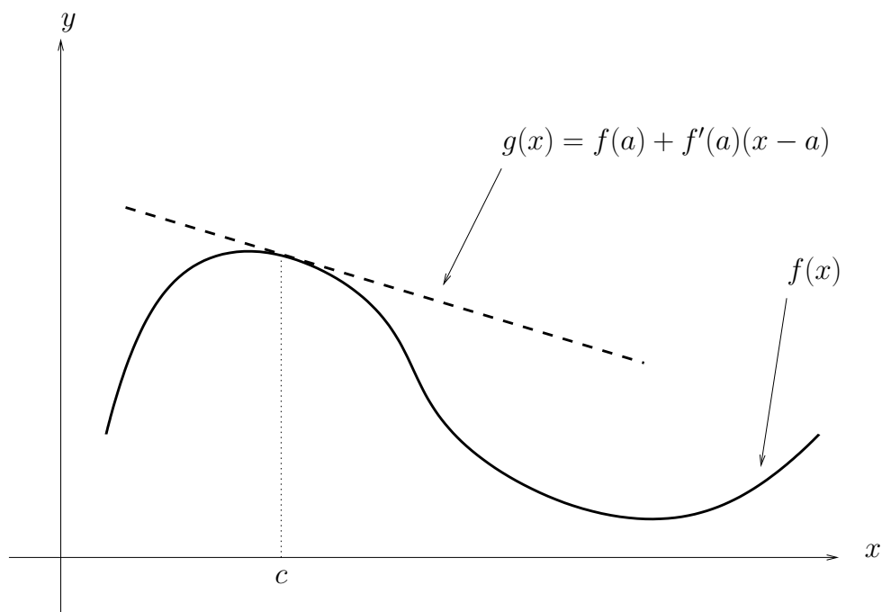
Figure 1: f diferenciável em a e a tangente ao gráfico de f em a .
